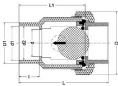
Шаровой обратный клапан с одним разборным окончанием ISR ХПВХ; с муфтовыми окончаниям, EPDM, IPS d20 (DN15)
