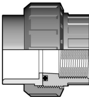
Муфта разборная с ВР ПВХ FIP 50x1 1/2
