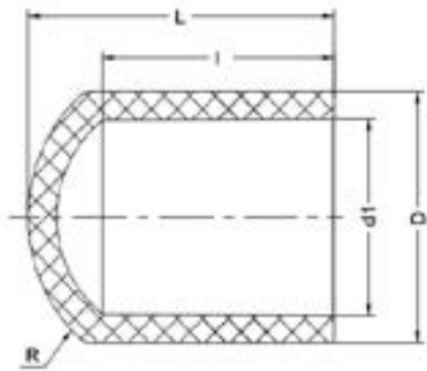
Заглушка ПВДФ для стыковой сварки d20 PN 16
