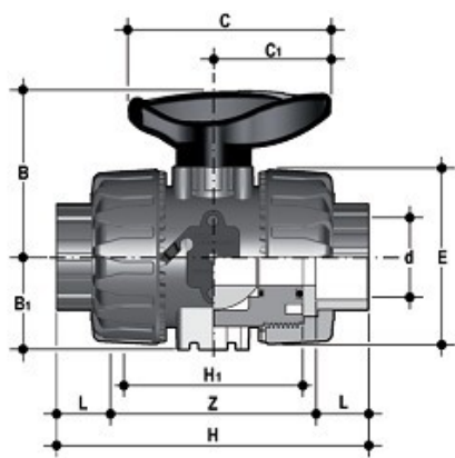
Шаровой кран ПВХ промышленного применения VKD с муфтовыми окончаниями, EPDM, FIP d90 (DN80)
