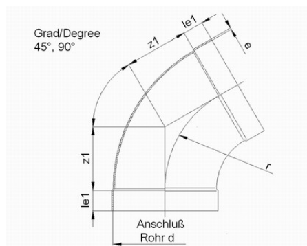
Изгиб 90° PPs d200
