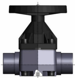
Мембранный клапан VMDC ХПВХ с втулочными окончаниями d110 (DN90)
