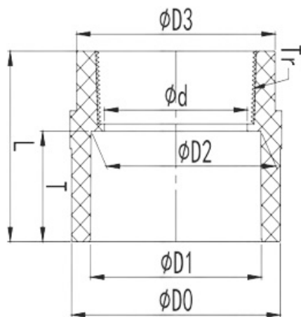
Муфта переходная с ВР ПВХ IPS 90x3"
