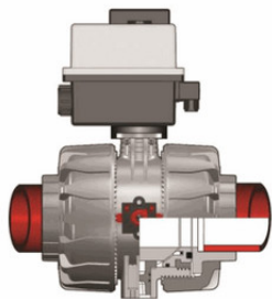
Шаровой кран VKD с эл.приводом 24V AC/DC, муфтовые окончания, DN65-100 (уплотнение EPDM) PP-H d75 (DN65)
