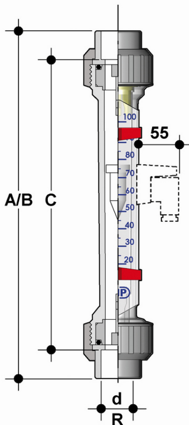
FS ротаметр для NaOH 30%; корпус: полисульфон d40
