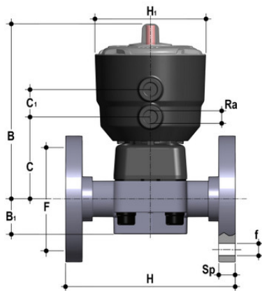
Мембранный клапан ПВХ с пневмоприводом, PN10, DK, EPDM, FIP d40 (DN32)
