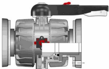
Шаровой кран VKD ПВДФ с фланцевыми окончаниями, DN65-100 d110
