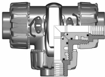
3-х ходовой шаровой кран ТКД ХПВХ с резьбовыми окончаниями, L-шар R1" (DN25)
