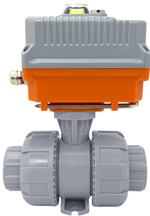
Шаровой кран IVKD ХПВХ с эл.приводом 24V DC, муфтовые окончания d50 (DN40)
