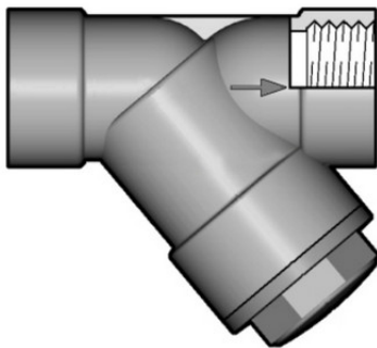
Грязевый фильтр из прозрачного ПВХ с резьбовыми окончаниями, EPDM, FIP R2½" (DN65)
