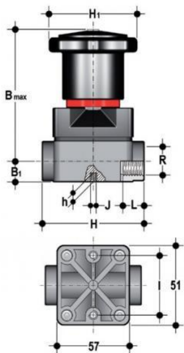
Компактный мембранный клапан CM ПВХФ с резьбовыми окончаниями R1/2" (DN15)
