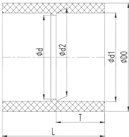
Муфта соединительная ПВХ IPS d63
