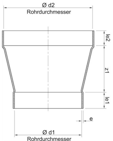
Муфта переходная PPs 250x160
