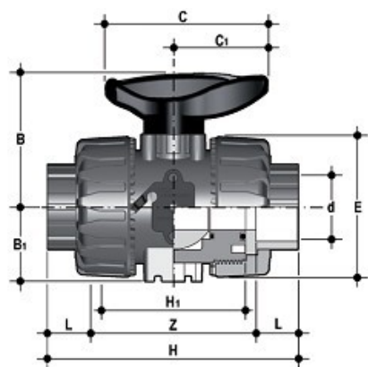
Шаровой кран ПВХ промышленного применения VKD с муфтовыми окончаниями, FKM, FIP d16 (DN10)
