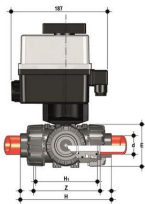
3-х ходовой шаровой кран ТКД с эл.приводом 90-240V, муфтовые окончания, Т-шар (уплотнение EPDM) PP-H d32 (DN25)
