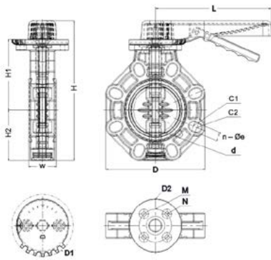
Затвор дисковый с рукояткой PP-H IPS d160 (DN150)
