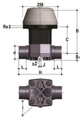
Мембранный клапан VM с пневмоприводом НЗ с втулочными окончаниями (уплотнение FKM/мембрана PTFE) PP-H d90 (DN80)
