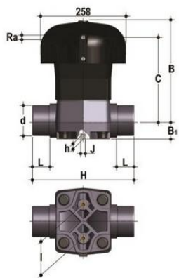
Мембранный клапан VM ХПВХ с пневмоприводом НО с втулочными окончаниями d90
