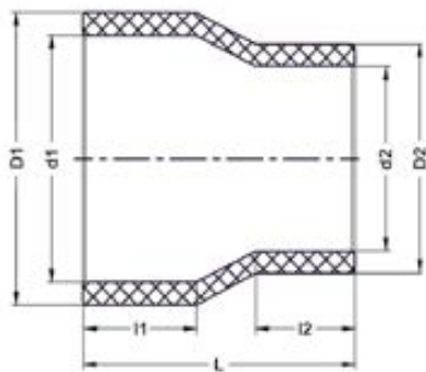
Муфта переходная для стыковой сварки PP-H IPS (Model B) 280x110 PN10
