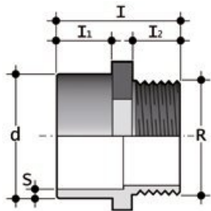
Адаптер с наружной резьбой PP-H FIP 40x1 SDR11 PN6
