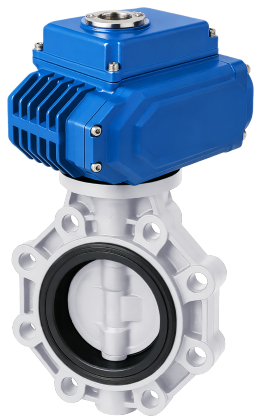
Дисковый затвор IFK ПВДФ с электрическим приводом 24V DC, EPDM, IPS d160 (DN150)
