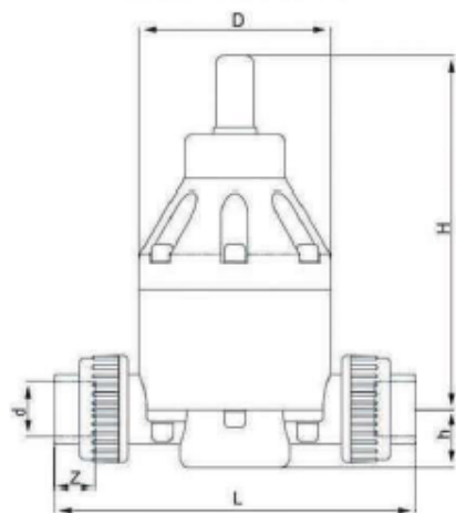
Клапан поддержания давления ПВХ с муфтовыми окончаниями, IPS d25 (DN20)
