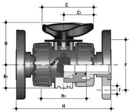
Шаровой кран ПВХ для регулирования потока VKR с фланцевыми окончаниями, FKM, FIP d32 (DN25)
