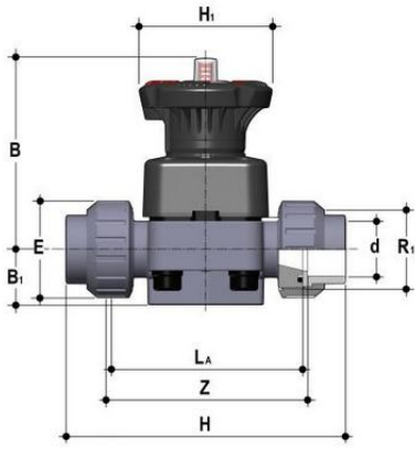
Мембранный клапан ДК ПВДФ с муфтовыми окончаниями d25 (DN20)
