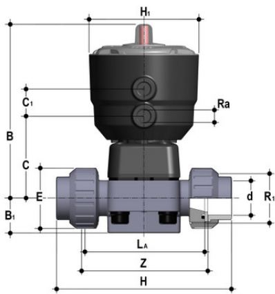
Мембранный клапан DK ПВХ с пневмоприводом НЗ, PN10, муфтовые окончания, EPDM, FIP d63 (DN50)
