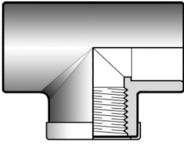
Тройник переходной с НР ПВХ FIP 50x1 1/2
