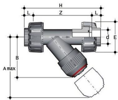
Грязевой фильтр RV ХПВХ с муфтовыми окончаниями d63 (DN50)
