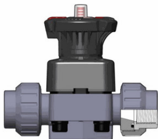
Мембранный клапан ДК ХПВХ с разборными резьбовыми окончаниями R1½" (DN40)
