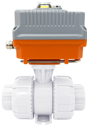
Шаровой кран IVKD ПВДФ с эл.приводом 24V DC, муфтовые окончания, FKM, IPS d20 (DN15)
