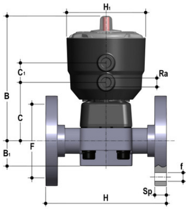
Мембранный клапан ДК ХПВХ с пневмоприводом НЗ, PN10 с фланцевыми окончаниями d32 (DN25)
