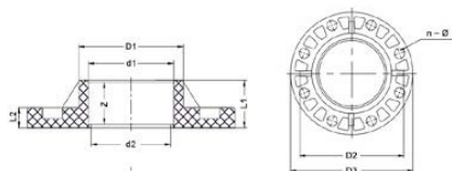
Жесткий фланец ХПВХ IPS (Model B) d630 PN10
