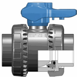
Шаровой кран ПВХ общего применения VEE; муфтовые окончания, EPDM, FIP d50 (DN40)
