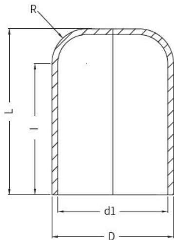
Заглушка ПВДФ для стыковой сварки d40 PN 16
