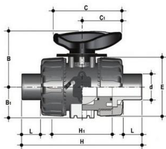
Шаровой кран для регулирования потока VKRDM с муфтовыми окончаниями (уплотнение FKM) PP-H d63 (DN50)
