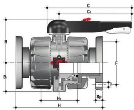
Шаровой кран промышленного применения VKD С фланцевыми окончаниями (уплотнение EPDM) PP-H d75 (DN65)
