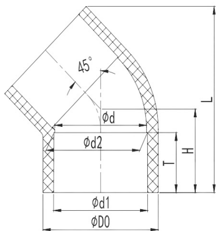
Отвод клеевой 45° ПВХ IPS d110
