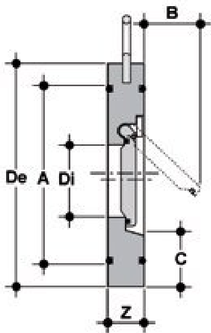
Межфланцевый обратный CROV ПВХ, EPDM, FIP d75 (DN65)
