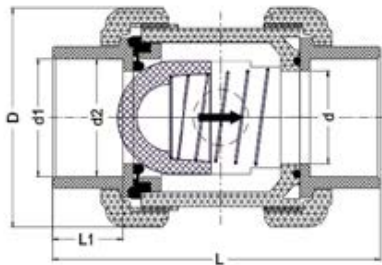
Пружинный обратный клапан ISSE ПБХ; с муфтовыми окончаниям, FKM, IPS d20 (DN15)
