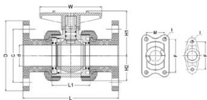
Кран шаровой промышленного применения с фланцевыми окончаниями PP-H IPS d25
