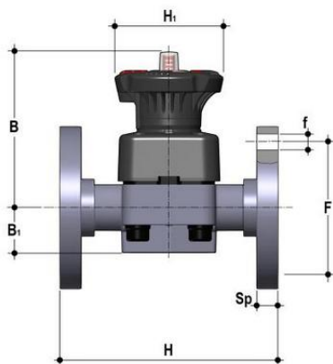
Мембранный клапан DK ХПВХ с фланцевыми окончаниями d50 (DN40)
