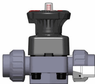
Мембранный клапан DKUIV PBX с разборными муфтовыми окончаниями, PTFE, FIP d25 (DN20)
