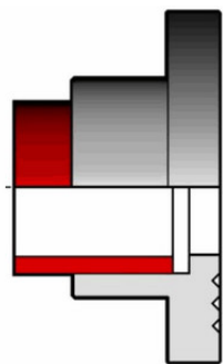
Бурт для раструбной сварки PP-H FIP d50 PN10
