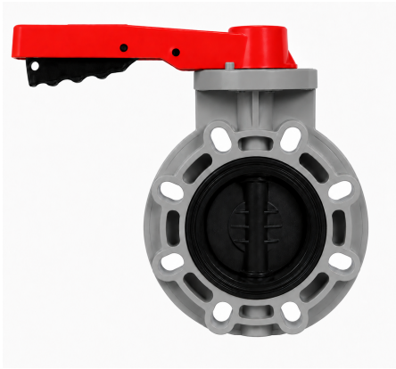
Затвор дисковый в корпусе FRPP (диск - НПВХ) с рукояткой промышленного применения FKM IPS 75 (DN65)
