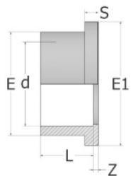
Бурт ХПВХ Comer d63 PN16
