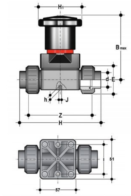
Компактный мембранный клапан CMUFV PBX с разборными муфтовыми окончаниями, EPDM, FIP d15 (DN15)
