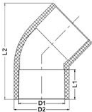
Отвод 45° ХПВХ IPS (Model A) d160 PN16
